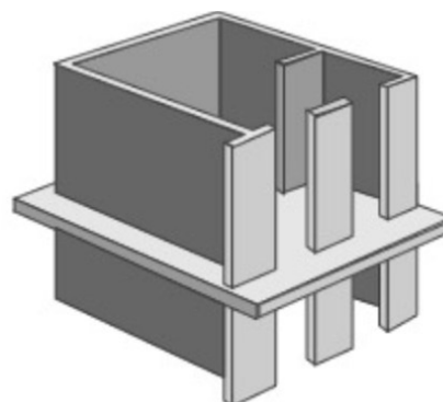
壁式構造
