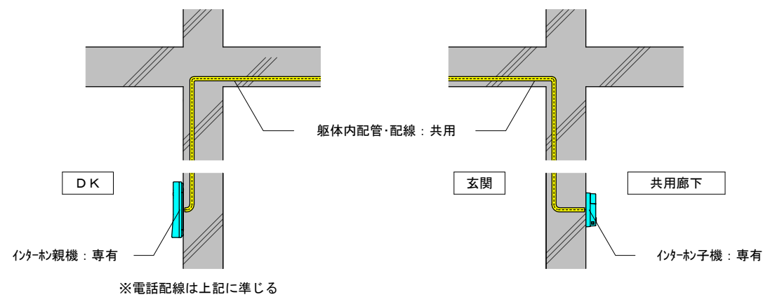
インターホン配線参考図 S=1:20
