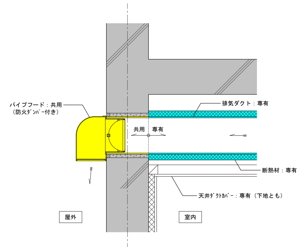
排気ダクト断面詳細図 S=1:10
