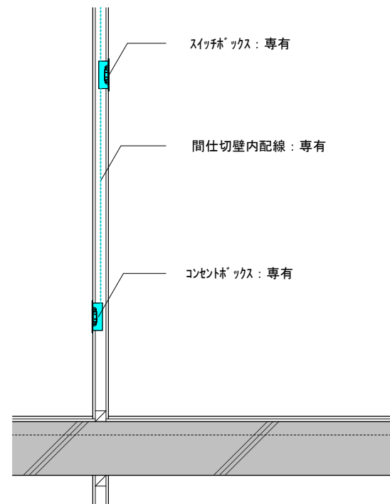
間仕切壁廻り配線参考図 S=1:20
